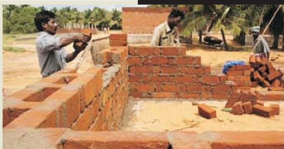
La Technique du « Rat-trap bond » permet une réduction de 30% d'utilisation de ciment et fers.
