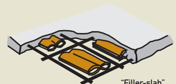
"Filler-slab"
